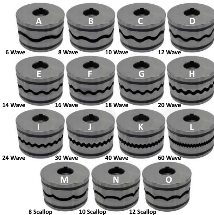
VI - 231 Bangle Pressing Die
